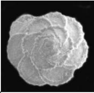
Globotruncana taille : entre 1mm et 0,25mm – photo fiche ECE
