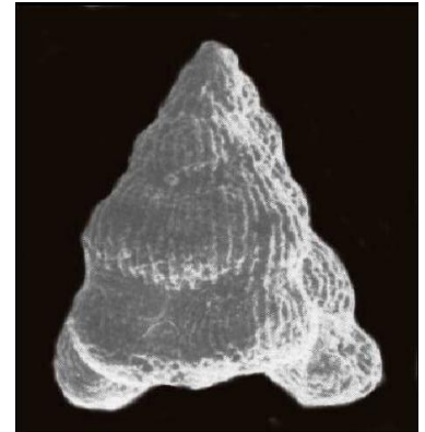
Heterohelix photo fiche ECE
